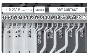
AUX 1 3 & 4 База (насос) или ультрафиолет (согласно модели)
