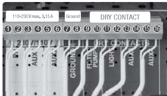
Фильтрационный насос Управление фильтрацией ⑨ & ⑩
